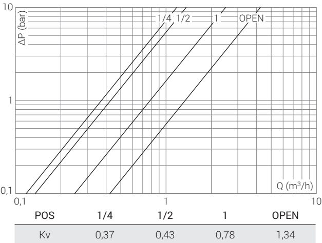
1/2" 0566 0526 Вентили прямые Heizkörperventile, Durchgangsform
