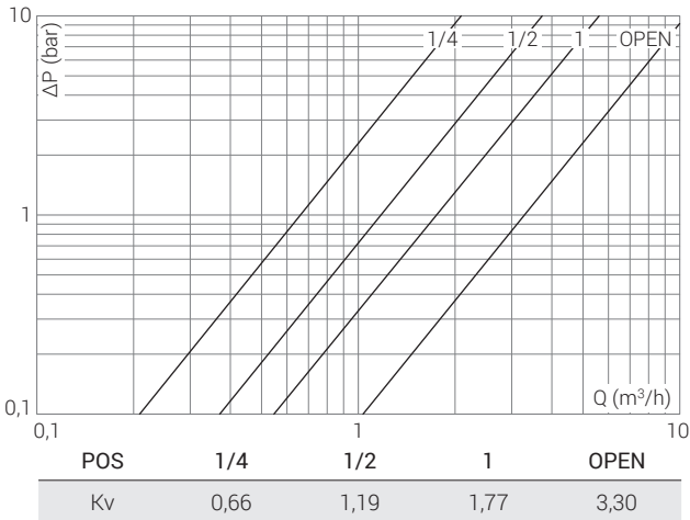
3/4" 0526 Вентили прямые Heizkörperventile, Durchgangsform
