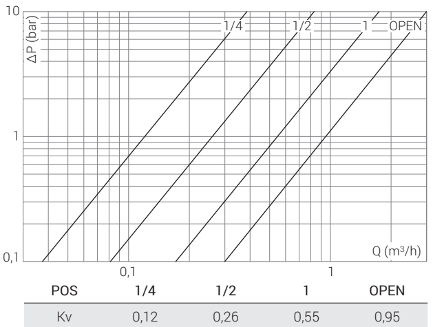
3/8" 0566 0526 Вентили прямые Heizkörperventile, Durchgangsform
