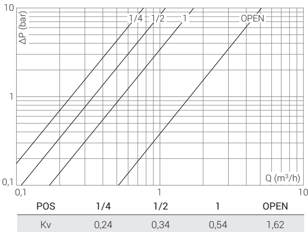
1/2" 0565 0525 Вентили угловые Heizkörperventile, Eckform
