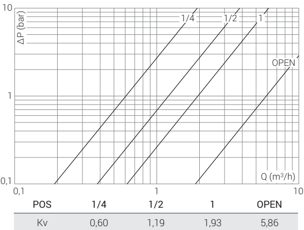
3/4" 0525 Вентили угловые Heizkörperventile, Eckform
